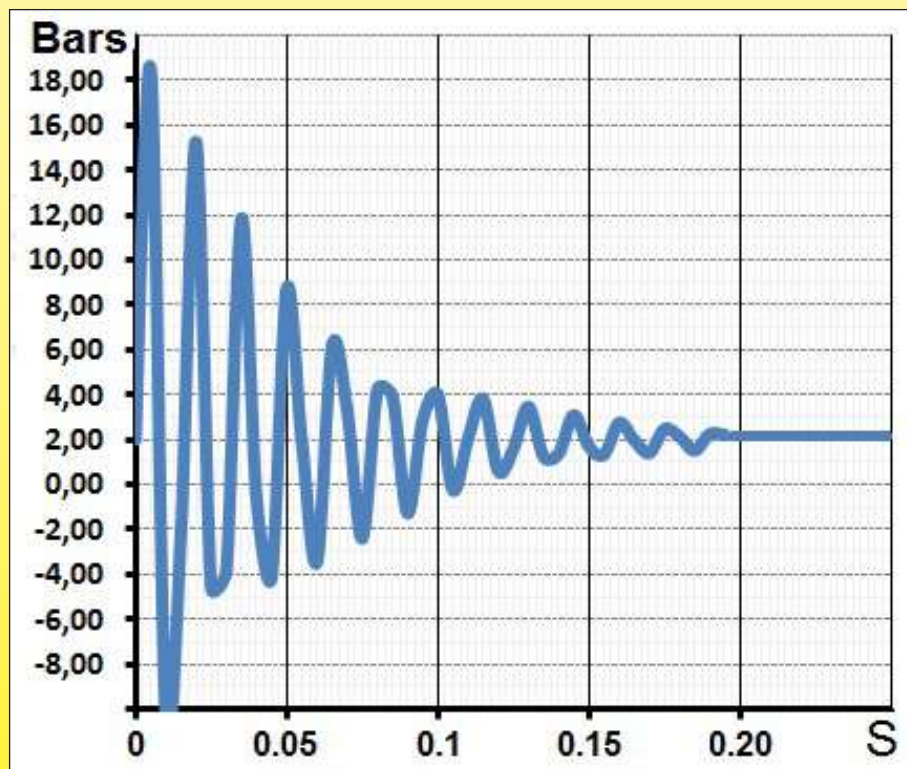
Forme typique de l'onde de choc lors d'un coup de béliér dans un réservoir diamètre 125mm, avec une pression du circuit de 2 bars, et une vitesse de circulation 0.5m/s dans la tuyauterie d'alimentation
