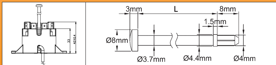
Rallonges de réarmement manuel
